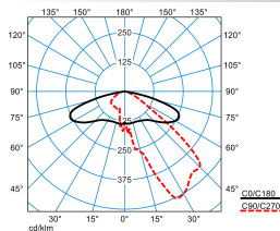
Publisca P2-AB2L/3200-740 4G1S TX047719 DIN 5040: A30 UTE: 1,00 G DLOR: 100 % ULOR: 0 % CEN Flux Code: 35 73 97 100 100
