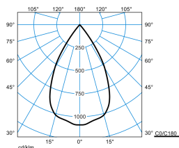
E-Line PRO 78 BV G2 RF-VFL 40-EC M39 ETDD 01 Blank
