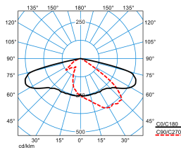
LnPlus 60-AB7L-LR/24000-740 18G1 ET (CLO end value)
