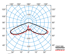
Publisca P2-RB6L-LRA/2200-740 3G1S ET (CLO end value)
