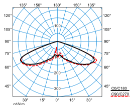
Publisca P2-RB6L-LRA/2200-740 3G1S ET (CLO initial value)
