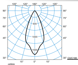
Faciella 08 RB1L/250-amber 1G1
