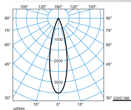
E-Line PRO 78 Lentyp L-MF 35-BF M54 ETDD 05 Blank
