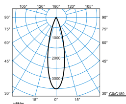
E-Line PRO 78 Lentyp L-MF 35-BF M54 ETDD 05 05
