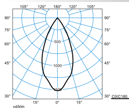
E-Line PRO 78 BV G2 RF-WFL 30-BF M54 ET 01 01
