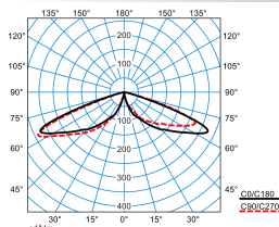
LTX P-RB6L-LRA/2600-740 3G1 ETDD
