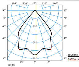
LPCV 3P2-ST L-W19 01 65-840 K04 ETDD 01
