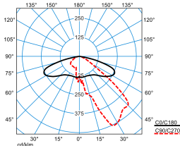
Publisca P2-AB2L-LR/3200-730 4G1S TX047755 DIN 5040: A30 UTE: 1,00 G DLOR: 100 % ULOR: 0 % CEN Flux Code: 35 73 97 100 100
