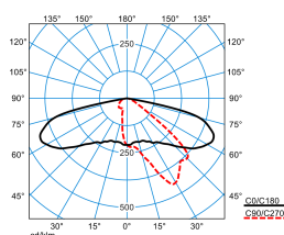
Cuvia40-AB2L4LR-S2-42-727-ET-CAE-26 (CLO end value)
