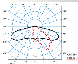
Cuvia40-AB2L4LR-S2-42-727-ET-CAE-26 (CLO initial value)
