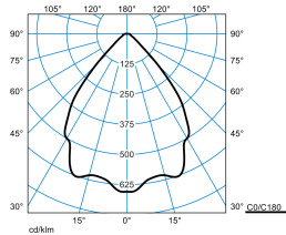
InperiaLP C05 HR22 1000-830 03 + DA-M 01
