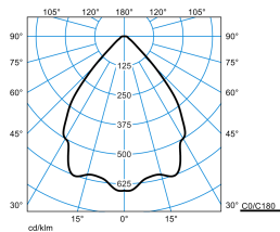
InperiaLP C05 HR22 1000-830 03 + DA-M 03
