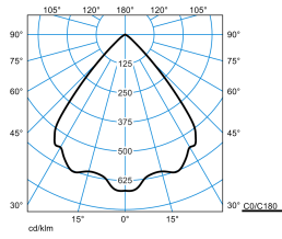
InperiaLP C05 HR22 1000-830 ET 03
