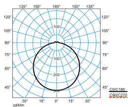
Olisq QWD3 DW 30-830 ET EB3 IK + Olisq QWD3 ZDR 1/2 05
