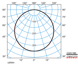
Olisq QWD3 DW 30-830 ET EB3 IK + Olisq QWD3 ZDR 1/1 01
