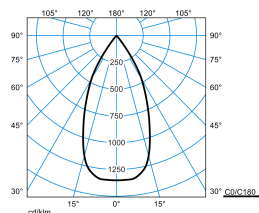
E-Line PRO 78 BV G2 RF-WFL 20-BF M54 ET 05 05
