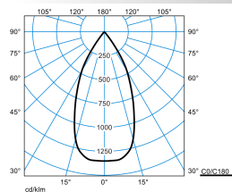
E-Line PRO 78 BV G2 RF-WFL 20-BF M54 ET 05 Blank
