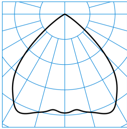
InperiaL G2 C07 HR22 1800-840 ET 03 ■ C0 - C180 TX769905
