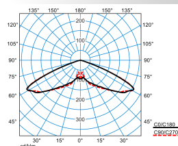
Publisca P1W-RB6L-LRA/3800-730 6G1S ET (CLO initial value)
