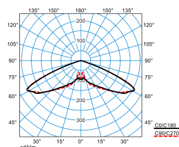
Publisca P1W-RB6L-LRA/3800-730 6G1S ET (CLO end value)
