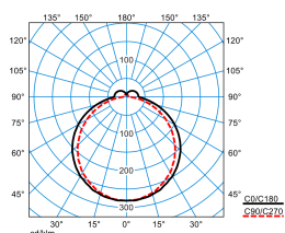
Olisq LWD1 DW 20-40/4/ML-840 ET IP54 IK (stage 4) TX564654
