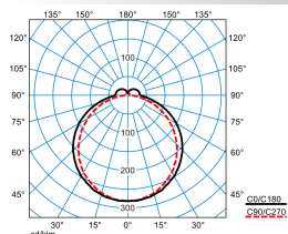
Olisq LWD1 DW 20-40/4/ML-840 ET IP54 IK (stage 1)
