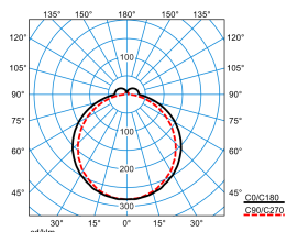
Olisq LWD1 DW 20-40/4/ML-840 ET IP54 IK (stage 3)
