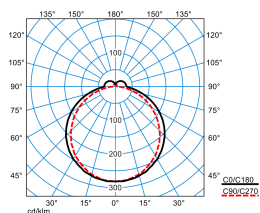
Olisq LWD1 DW 20-40/4/ML-840 ET IP54 IK (stage 4)
