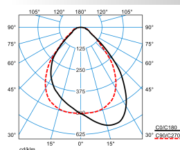
ArimoFit G2 M57 P-WW 42-8TW ETDD8 (DWW)
