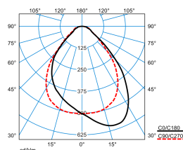
ArimoFit G2 M57 P-WW 42-8TW ETDD8 (DSU)
