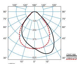
ArimoFit G2 M57 P-WW 42-8TW ETDD8 (DCW)
