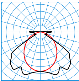
Nextrema G3 B 40-840 ET TWP TX768184
