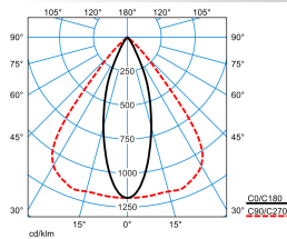
YVTW 3P L-OVL 30-830 M33 ET 01 (LEO1)
