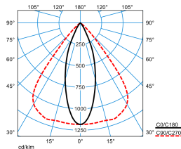
YVTW 3P L-OVL 30-830 M33 ET 01
