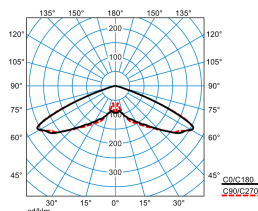
Publisca P1W-RB6L-LR/3800-740 6G1S ET (CLO end value)
