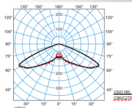
Publisca P1W-RB6L-LR/3800-740 6G1S ET (CLO initial value)
