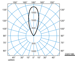
Altigo G2 60 WO RB17L/2000-830 1G1P + VE IP66 24V DC 250W TX120511
