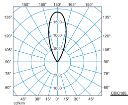
Altigo G2 60 WO RB17L/2000-830 1G1P + VE IP66 24V DC 130W TX120449
