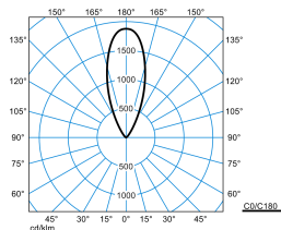
Altigo G2 60 WO RB17L/2000-830 1G1P + VE IP66 24V DC 60W TX120475
