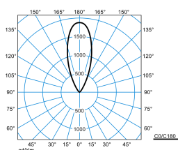
Altigo G2 60 WO RB17L/2000-830 1G1P + G2 VE IP66 24V DC 30W
