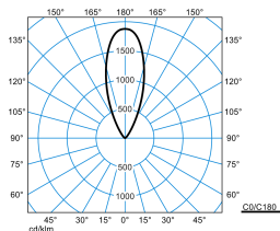
Altigo G2 60 WO RB17L/2000-830 1G1P + VE IP66 24V DC 250W
