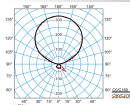
Luceos S-T PAW-IL 300-840 ETDI 03+LLWP (LEO1)
