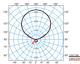
Luceos S-T PAW-IL 300-840 ETDI 03+LLWP (LEO2)
