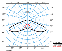
Publisca P2-RB6L-LRA/1650-730 2G1S ET (CLO initial value)
