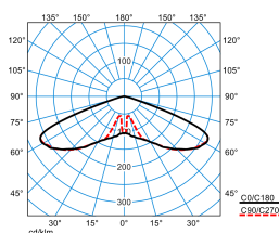
Publisca P2-RB6L-LRA/1650-730 2G1S ET (CLO end value)
