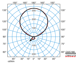
Luceos S-U PAW-IL 170-840 ETDS 03 (LEO1) TX830364
