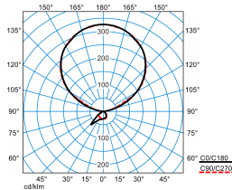
Luceos S-U PAW-IL 170-840 ETDS 03 (LEO2) TX830365
