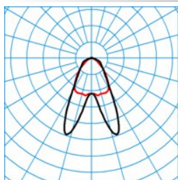
ELINE HE+ LDAN100 830 L225 1 20 ■ C0 - C180
