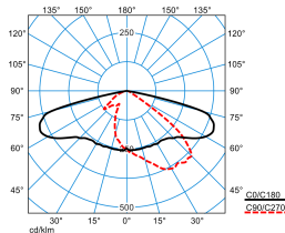
LnPlus 60-AB7L-SLR1/26000-722 24G1 ET (CLO initial value)
