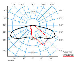
LIQ 50N-AB2L-LR/135/165/200-740 2G1 ET (CLO end value)
