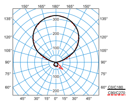
Luceos S-T PAW-IL 300-830 ETDI 03+LLWP (LEO1)
