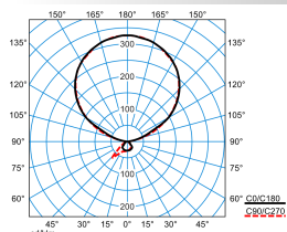
Luceos S-T PAW-IL 300-830 ETDI 03+LLWP (LEO2)
