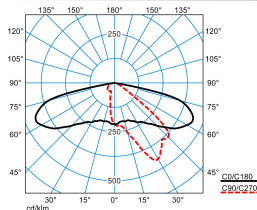
Publisca P3-AB2L-SLR3/4200-740 4G1 ET (CLO initial value)
