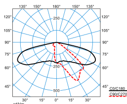
Publisca P3-AB2L-SLR3/4200-740 4G1 ET (CLO end value)
