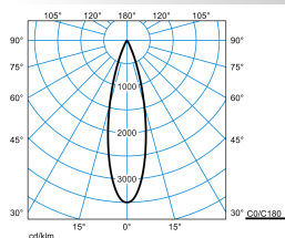
7651 LentyP L-MF 20-EC M39 ET 01 (225)
