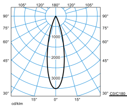
7651 Lentyp L-MF 20-EC M39 ET 01 (150)
