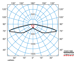
Publisca P3-SB3L-LRA/1800-730 2G1 ET (CLO end value)
