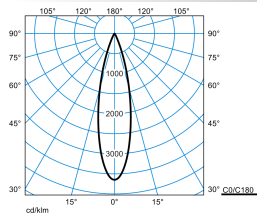
7651 LentyP L-MF 30-BC M49 ETDD 05 (150)
