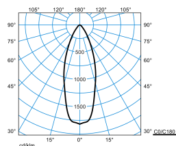
Amatris RC1 SRRFL 4/8/ML-9MC ETDD 05 (stage 5)
