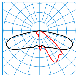
Publisca P1-AB2L-LR/2600-730 3G1S TX047523 ■ C0 - C180 ■ C90 - C270 DIN 5040: A30 UTE: 1,00 l DLOR: 100 % ULOR: 0 % CEN Flux Code: 34 71 96 100 100
