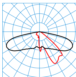
Publisca P1-AB2L-LR/2600-730 3G1S ET (CLO initial value) TX300848 ■ C0 - C180 ■ C90 - C270 DIN 5040: A30 UTE: 1,00 l DLOR: 100 % ULOR: 0 % CEN Flux Code: 34 71 96 100 100
