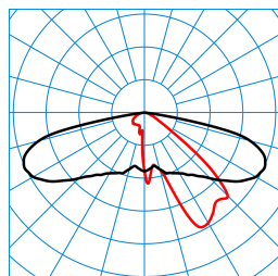
Publisca P1-AB2L-LR/2600-730 3G1S ET (CLO end value) TX301115 ■ C0 - C180 ■ C90 - C270 DIN 5040: A30 UTE: 1,00 l DLOR: 100 % ULOR: 0 % CEN Flux Code: 34 71 96 100 100
