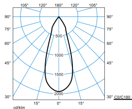
E-Line PRO 78 BV G2 RF-FL 50-840 M35 ET 01 Blank
