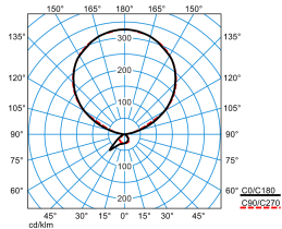
Luceos S-U PAW-IL 170-840 ETDS 05 (LEO2) TX830366
