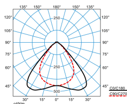
7850 PW2255-120 ML 840 L225 10 50
