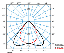
7850 PW2255-120 ML 840 L225 12 50
