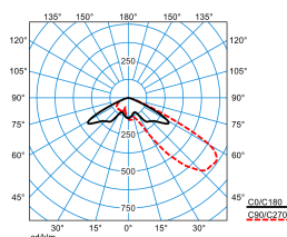
LnPlus 60-AM19L-SLR1/26000-730 24G1 ET (CLO end value)
