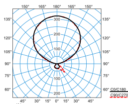
Luceos S G2 PAW-IL 150-8TW ETDI 03+LLWP (DSU)
