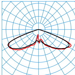
Publisca P2-RB6L-LRA/2600-740 3G1S TX047900 ■ C0 - C180 ■ C90 - C270 DIN 5040: A20 UTE: 1,00 J DLOR: 100 % ULOR: 0 % CEN Flux Code: 20 57 98 100 100
