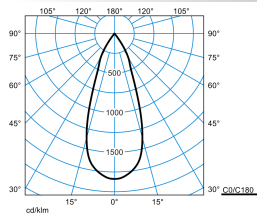
SisC 2Z RF-FL 2x30-830 M33 ET 01
