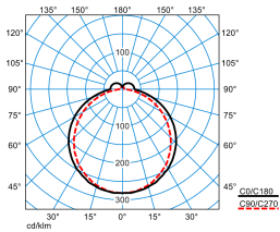
Olisq LWD2 DW 60-830 ET IP54 TX375589
