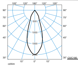
E-Line PRO 78 BV G2 RF-FL 30-BC M49 ETDD 05 Blank
