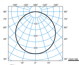
Olisq RWD2 DW 14-40/4/ML-840 ET + Olisq RWD2 ZDR 1/1 03 (stage 3)
