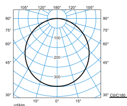
Olisq RWD2 DW 14-40/4/ML-840 ET + Olisq RWD2 ZDR 1/1 01 (stage 4)
