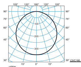
Olisq RWD2 DW 14-40/4/ML-840 ET + Olisq RWD2 ZDR 1/1 05 (stage 3)
