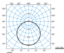
Olisq RWD2 DW 14-40/4/ML-840 ET + Olisq RWD2 ZDR 1/2 05 (stage 2)
