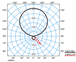
Luceos S BS G3 PAW-IL 125-830 ETDD FT 01
