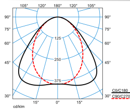
Cflex H1-E B 5500-840 ETDD EB3 I2
