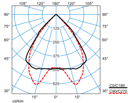
SFlow C3-L MRX LED4000-840 ETDD LLWM 01 TX771995
