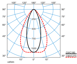
E-Line PRO 78IP50 MironaF T 130-840 ETDD L150 01 01 (LEO2)
