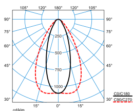
E-Line PRO 78IP50 MironaF T 130-840 ETDD L150 01 01 IP50 (LEO2)
