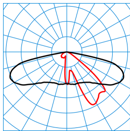
Publisca P2-AB2L/1800-730 2G1S TX047706 ■ C0 - C180 ■ C90 - C270 DIN 5040: A30 UTE: 1,00 G DLOR: 100 % ULOR: 0 % CEN Flux Code: 34 70 96 100 100
